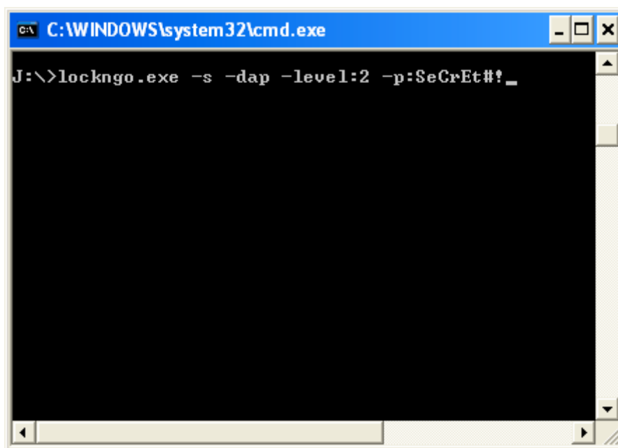
Рисунок 9: Командная строка
